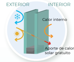
DETALLE DE CARPINTERÍA DOBLE*
