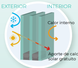
DETALLE DE CARPINTERÍA TRIPLE*
